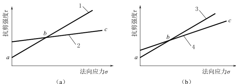
1—有效强度包线 CD；2—不排水剪总强度包线 UU； 3—有效强度包线 CD；4—固结不排水剪总强度包线 CU
