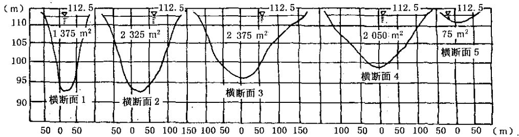
b) 库区横断面图
