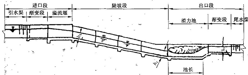
a) 甲-甲剖面
