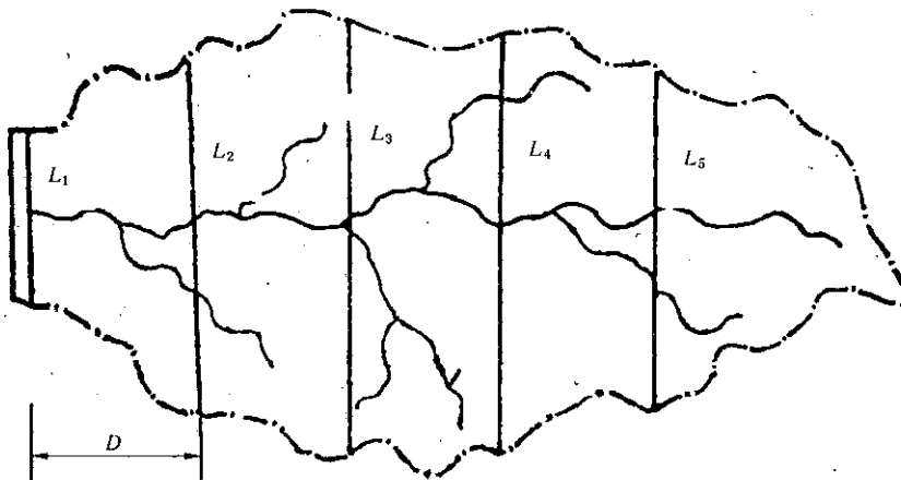
图 A.1 集中面积梯形计算法
