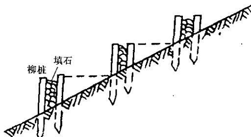
图 5 柳谷坊示意图
