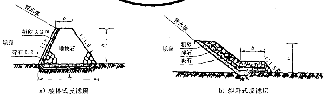
图 10 反滤体两种形式示意图
