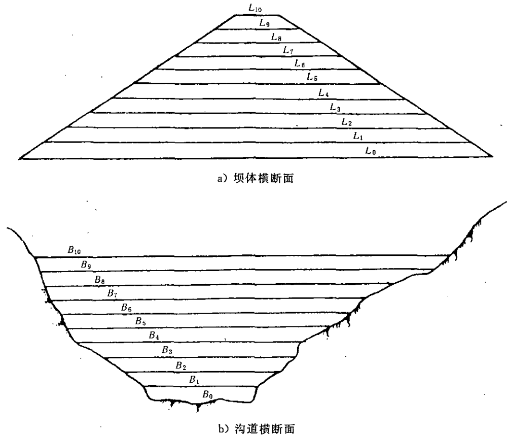
图 C.1 坝体土方计算简易长宽相乘法
