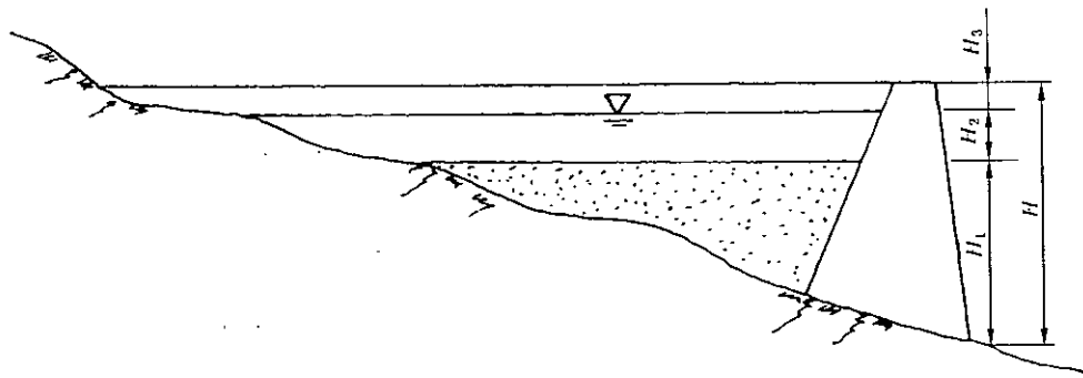
图7 坝高组成示意图
