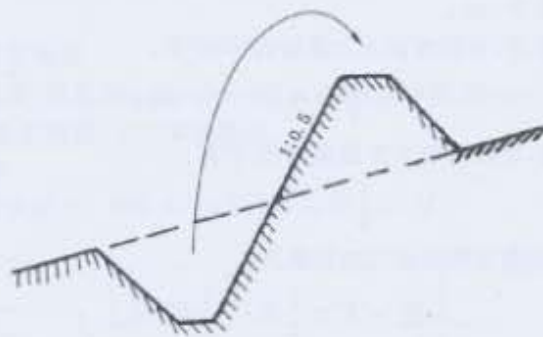
图 4 坡式梯田断面
