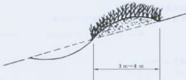
图 5 草带(或灌木带)坡式梯田
