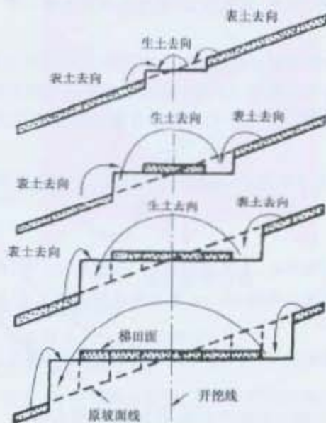
图7 表土逐行置换法
